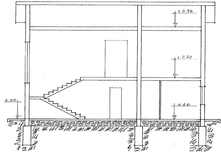
SEZIONE A-B
